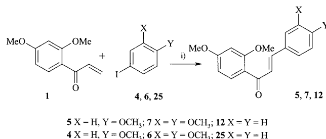
Scheme 1. i) \text{Pd}(\text{OAc})_2 , \text{Ph}_3\text{P} , \text{CH}_3\text{CN} , \text{Et}_3\text{N} , reflux
